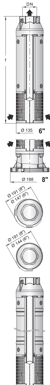
Collare speciale di rinforzo da 6SDX(L) 65/27
